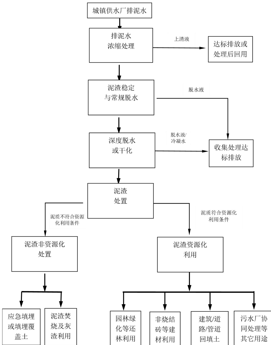
图 A 城镇供水厂泥渣处理处置与资源化利用技术路线
